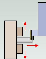
Die Futterbacken sind geöffnet und der Stangengreifer zieht die Stange auf die neue Bearbeitungsposition
